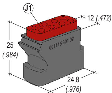
Taille 16 Size 16 8 Contacts (13 A) Masse : 12,20 g. Weight : 0,026 lbs
