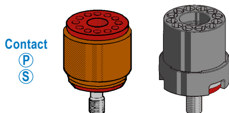
Module de masse circulaire Circular grounding module
